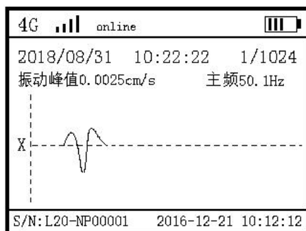
波形预览
